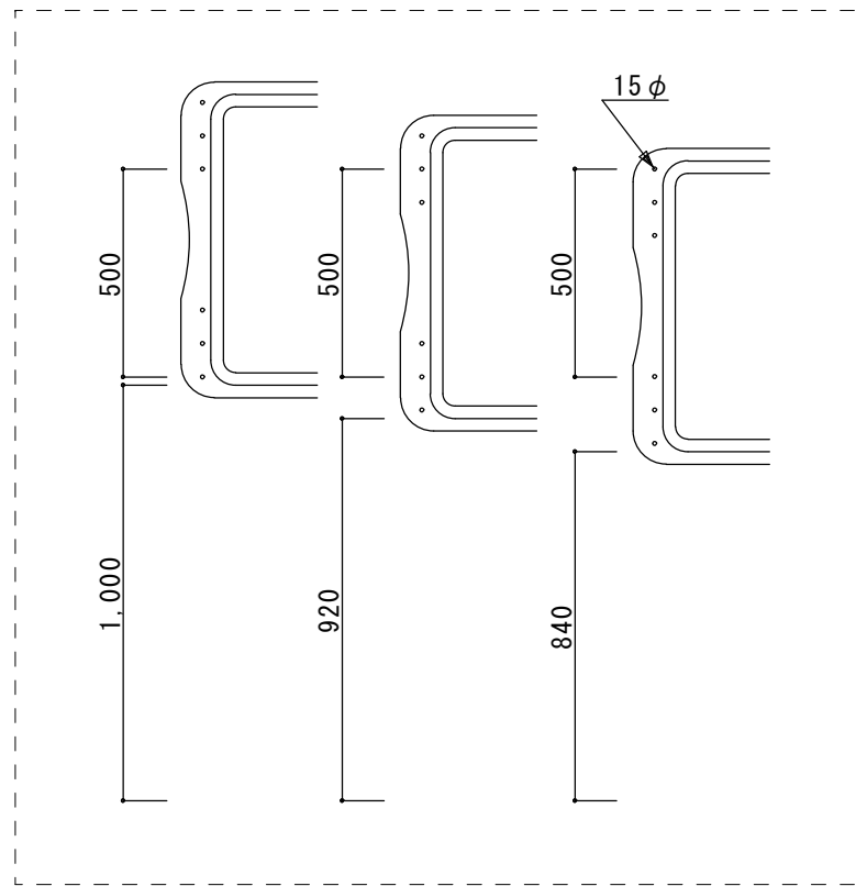
~ 脚取付位置 落差表 ~
